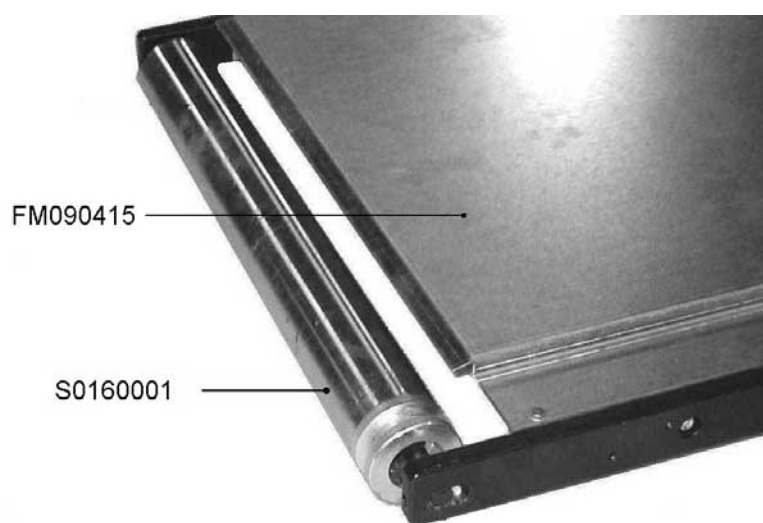
Lato uscita / Outlet side
