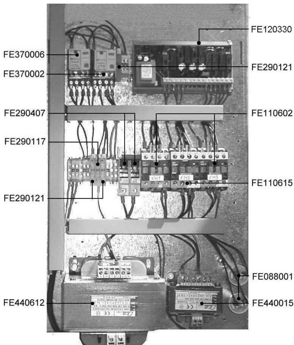
Cassetto elettrico / Wiring box
